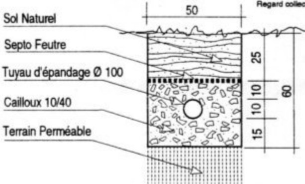
Détail "A" Éch.: 1/20
